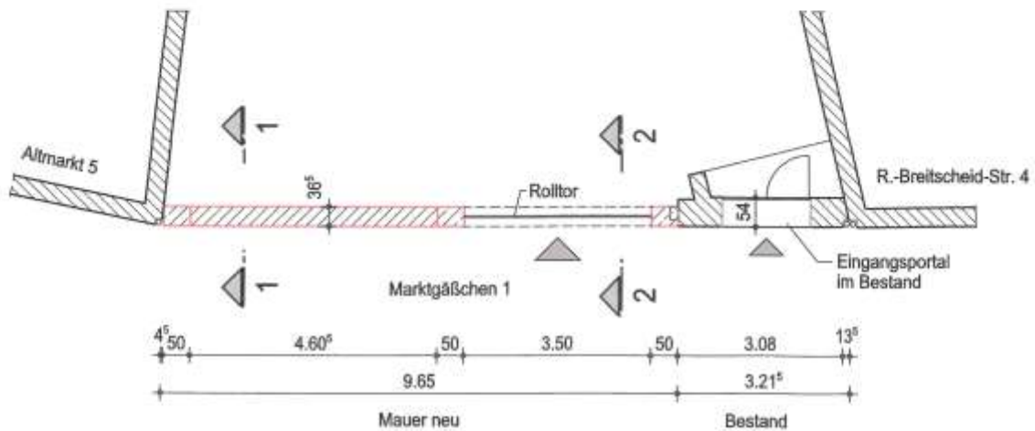
N GRUNDRISS
