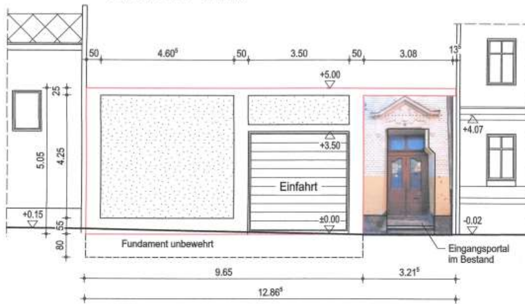
ANSICHT M 1:100
