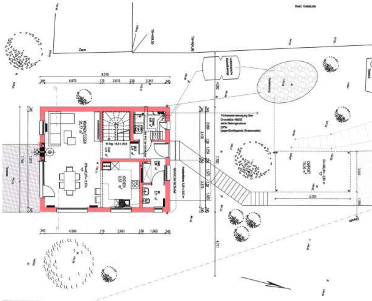
Auszug Grundriss Erdgeschoss zum Bauantrag
