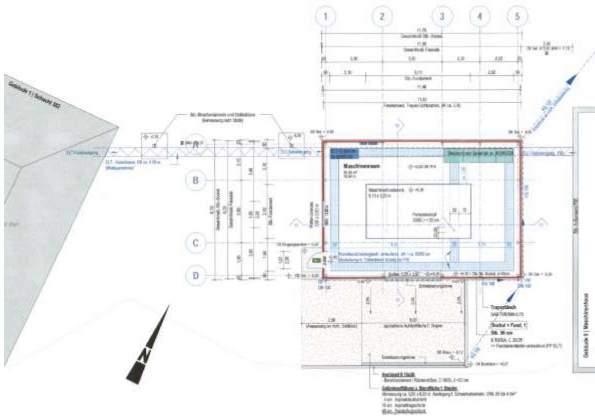
Auszug Grundriss zum Bauantrag
