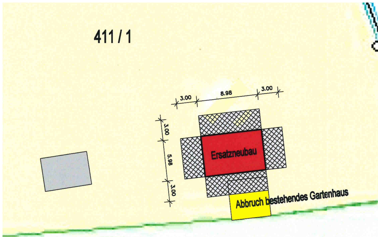
Auszug Lageplan zum Bauantrag vom 01.12.2022
