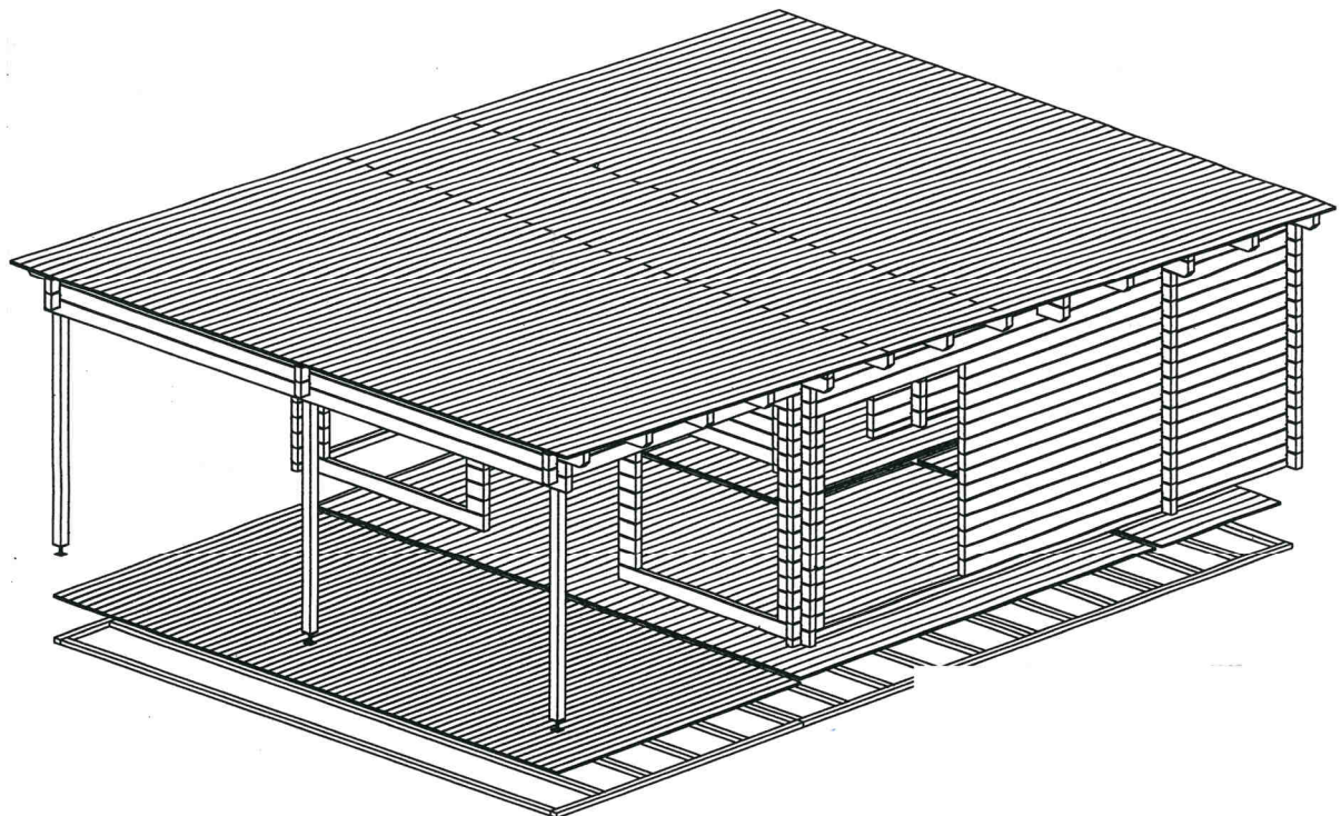
Isometrie geplante Laube
